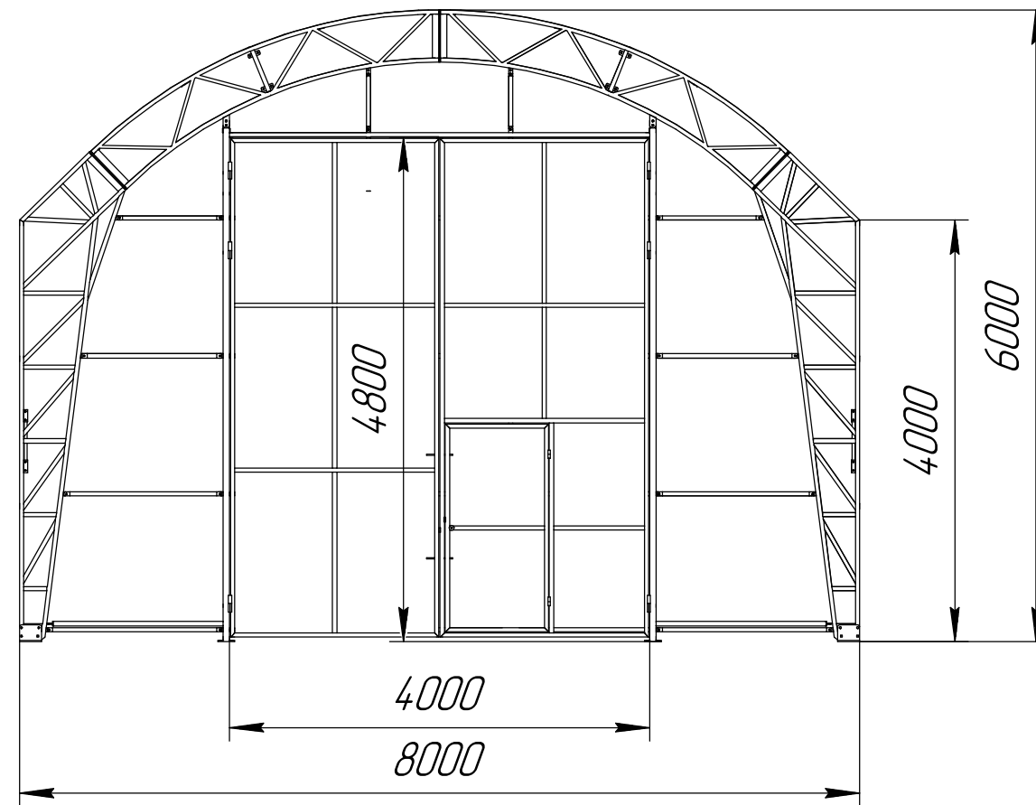
Ангар каркасный на стойках с тентовым укрытием 8х14х4(6) м.
