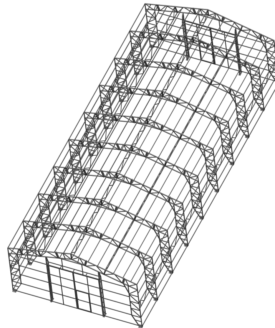
Ангар каркасный на стойках с тентовым укрытием 10х24х4,6(6,0) м.
